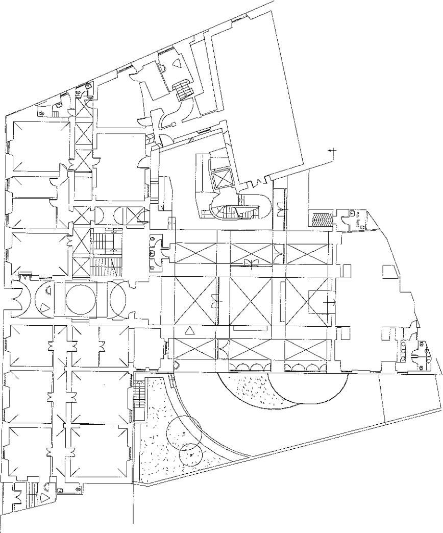
PALAZZO MUNICIPALE STATO ATTUALE PIANO TERRA SCALE 1:100
