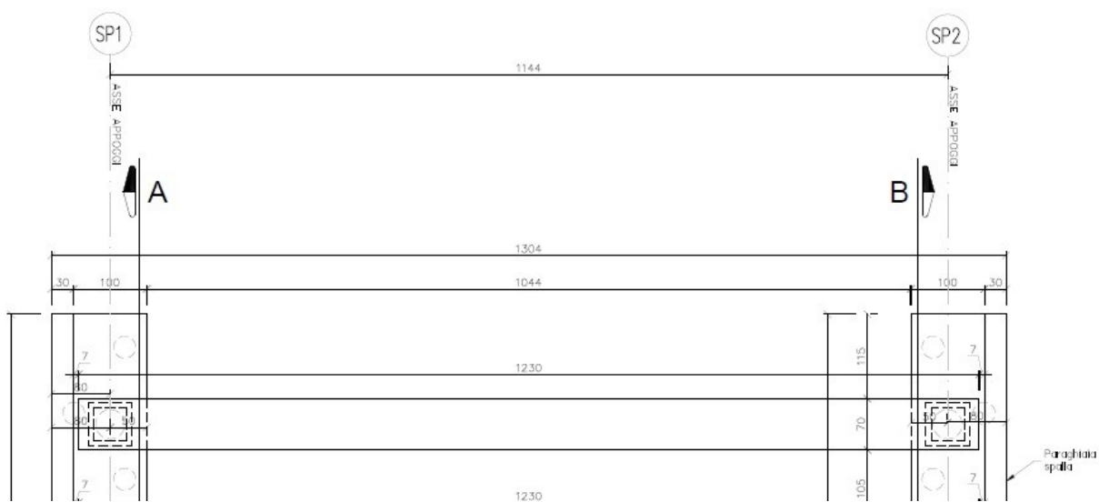
PIANTA SUPERIORE SCALA 1:50
