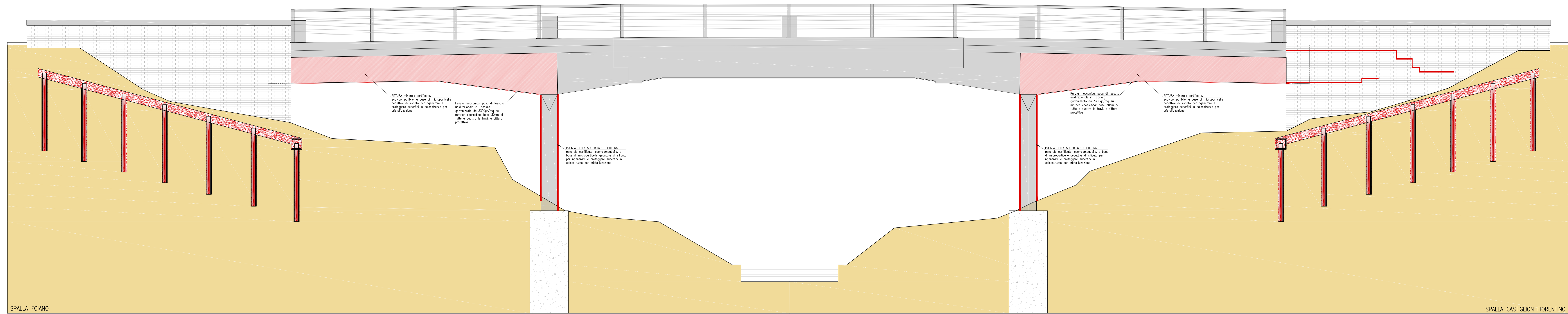
PROSPETTO LATERALE DELL'OPERA SCALA 1:50
