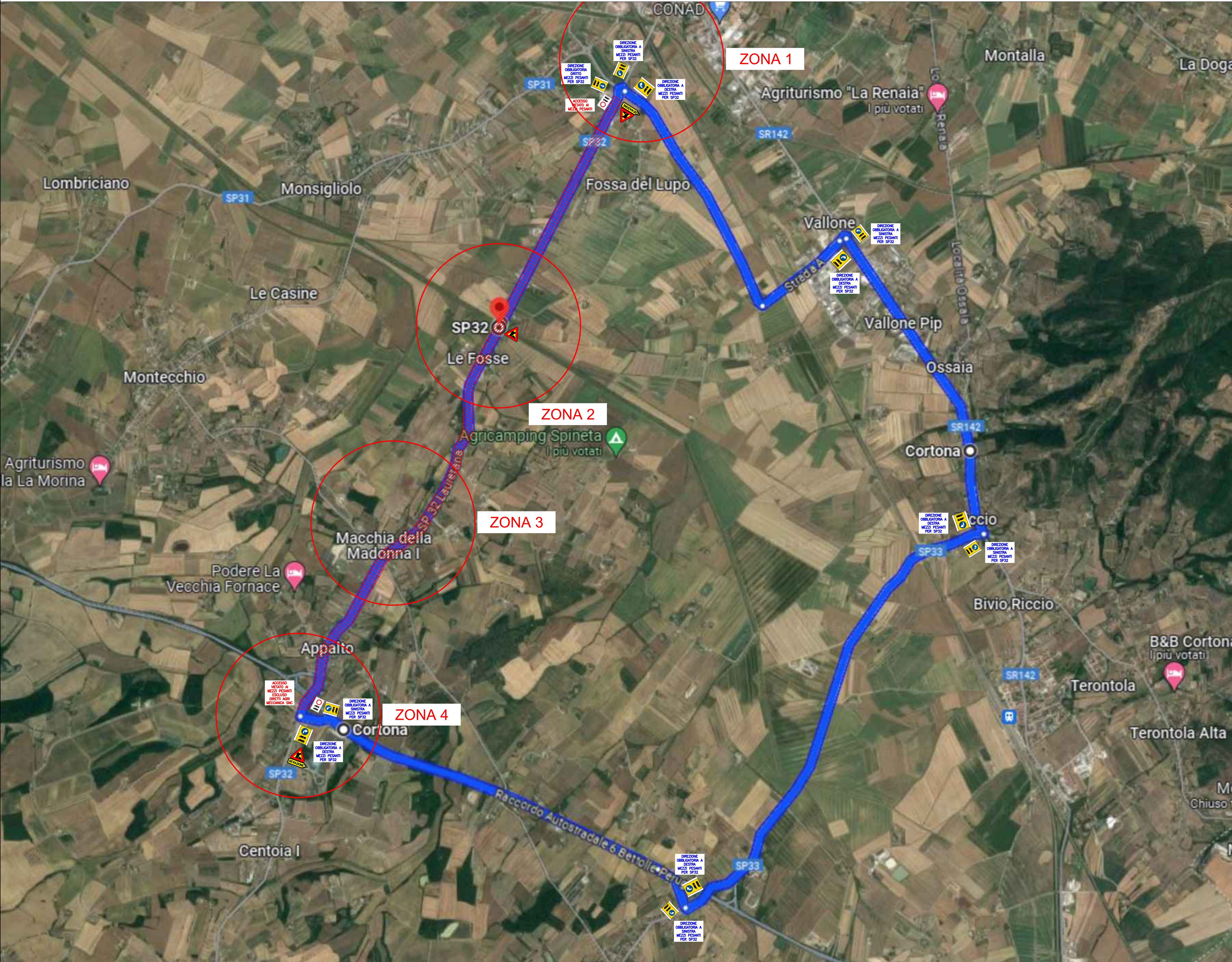
VIABILITA' ALTERNATIVA MEZZI PESANTI DURANTE L'ESECUZIONE DEI LAVORI
