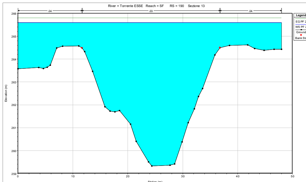
Fig. 13 Sezione 13 - RS=190.
