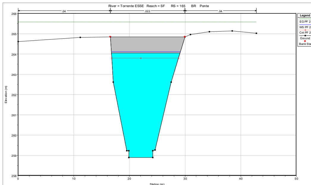
Fig. 16 Sezione in corrispondenza al ponte sulla S.P.25
