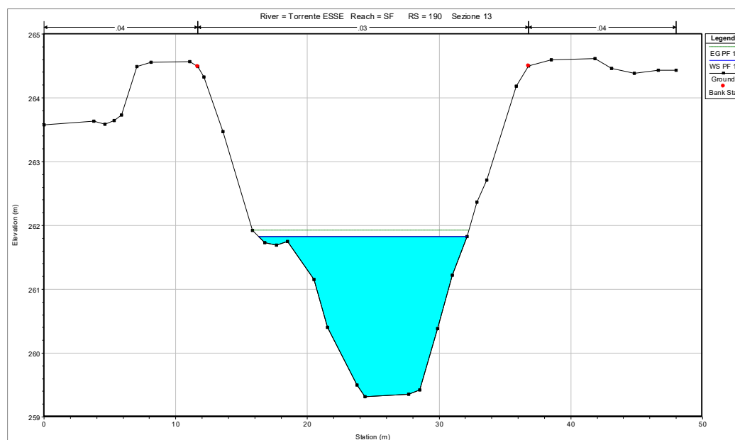
Fig. 7 – Sezione 13 RS=190.
