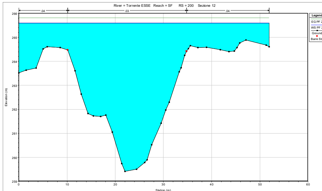
Fig. 12 Sezione 18 - RS=200.
