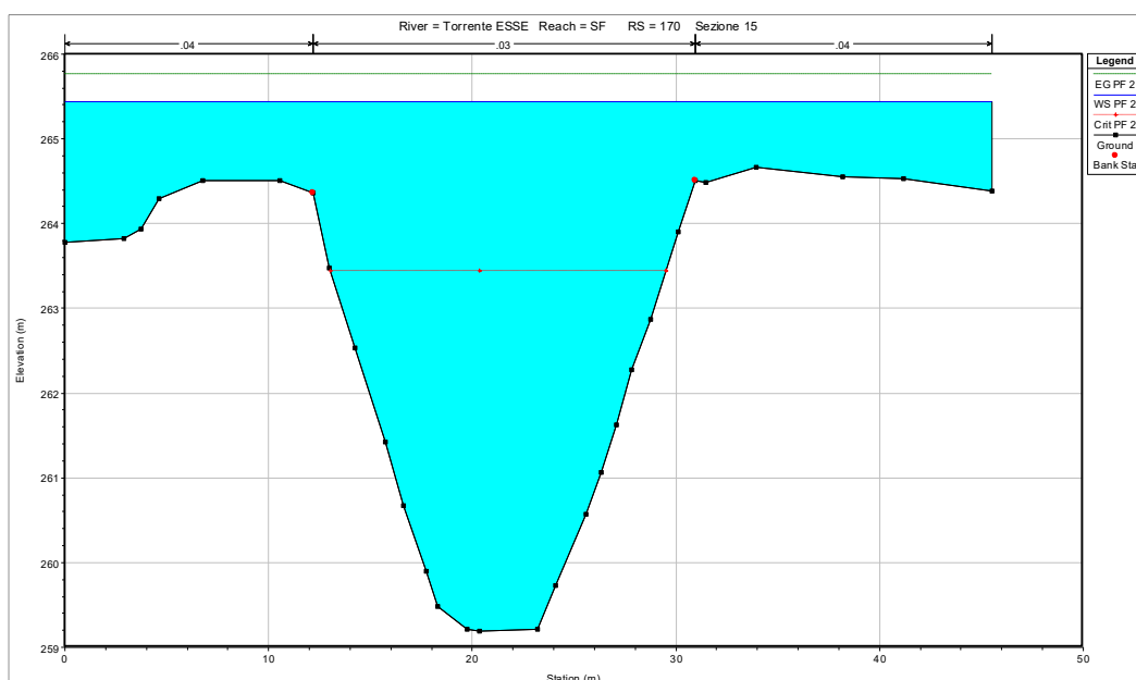
Fig. 15 Sezione 15 - RS=170.
