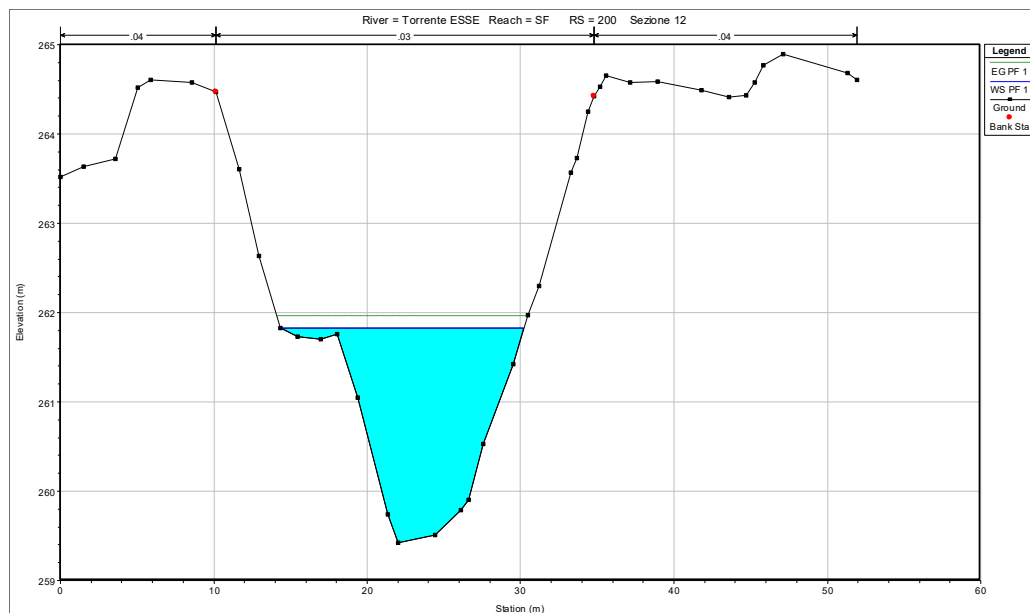
Fig. 6 – Sezione 12 RS=200.
