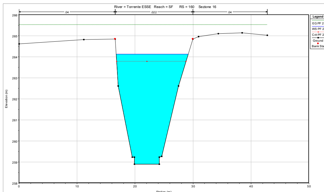
Fig. 17 Sezione 16 - RS=160.
