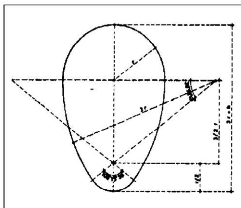
FIG. 21 - Collettori ovoidali. Sezione classica 2r - 3r
