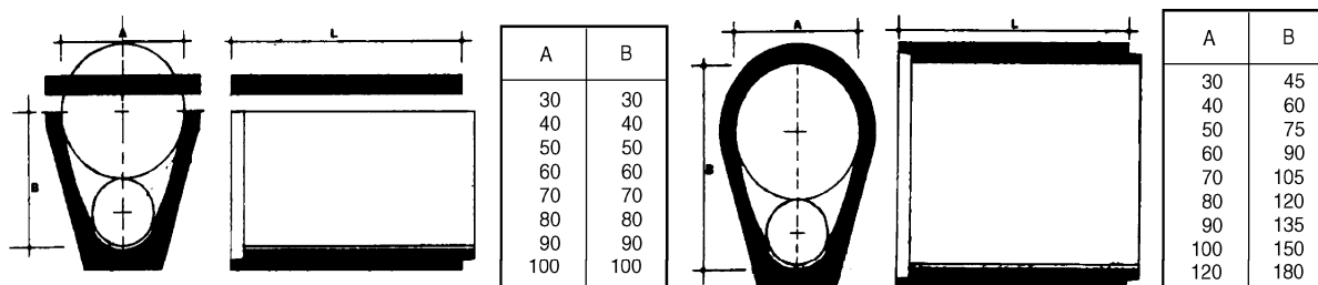
FIG. 22 - Condotti semiovoidali e ovoidali prefabbricati. Dimensioni indicative
