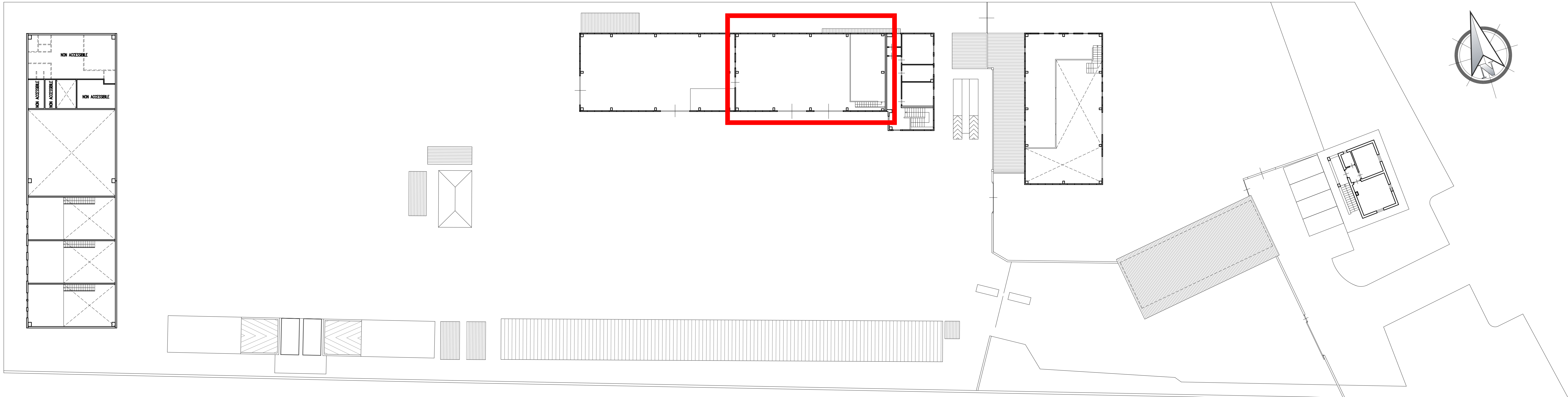
6 PLANIMETRIA GENERALE AUTOPARCO DELLA PROVINCIA DI AREZZO - PIANO PRIMO CON INDICAZIONE DELL'EDIFICIO OGGETTO DEI LAVORI DI RIMOZIONE E BONIFICA AMIANTO A01 Scala 1:200
